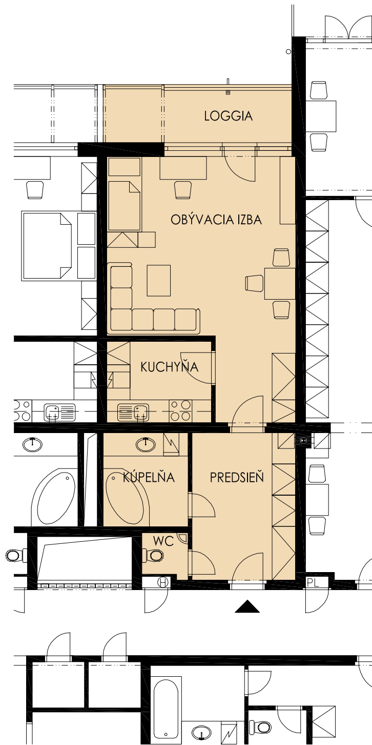
PÔDORYS, M 1:100
